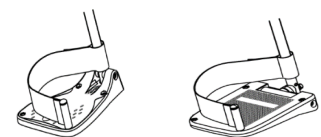
Fußplatte fest Fußplatte verstellbar für festes Beinstützenoberteil
