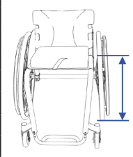
Sitzhöhe hinten gemessen von Rollstuhl Oberkannte Sitzrohr hinten bis Boden.
